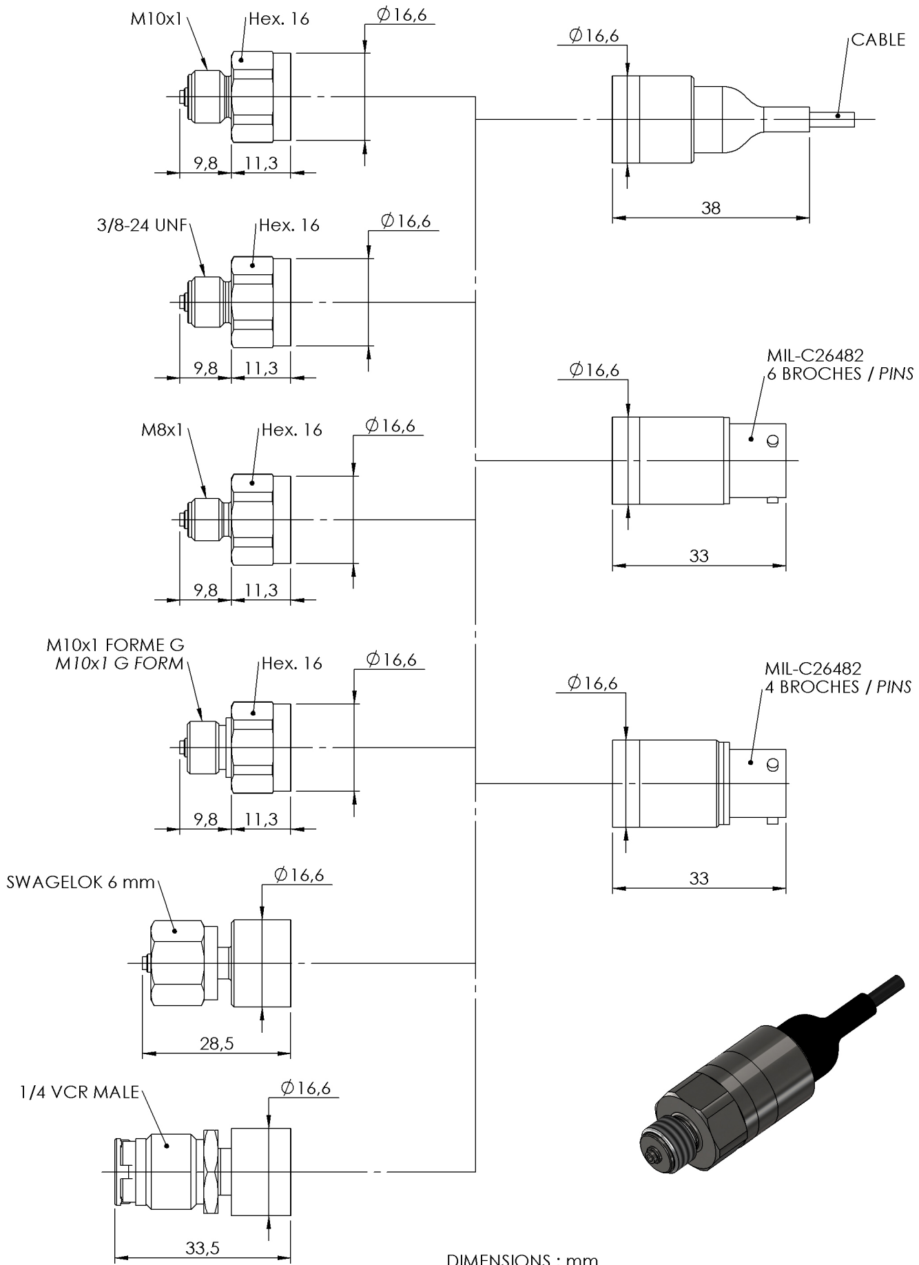
DIMENSIONS : mm
